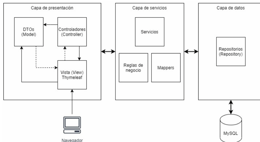
Fig. 6. Diagrama de arquitectura de AQUA.
